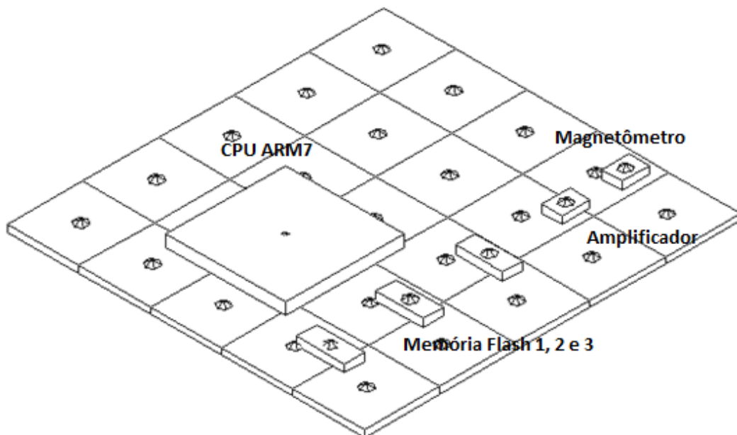
Figura 12: Modelo geométrico do Subsistema de Computador de Bordo
